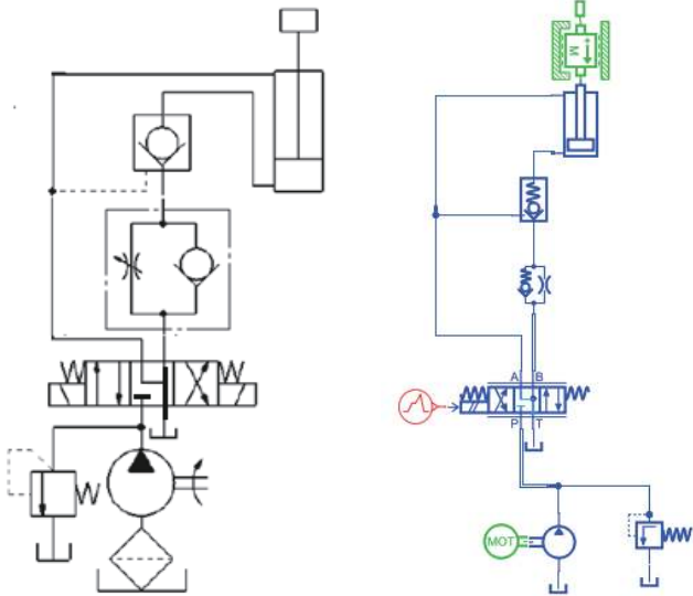
图5 采用液控单向阀的平衡回路 图6 平衡回路 AMESim 建模
