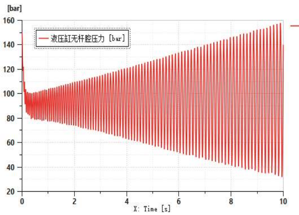
图7 液压缸无杆腔压力 1
