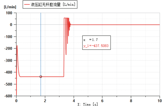
图 4 液压无杆腔流量
