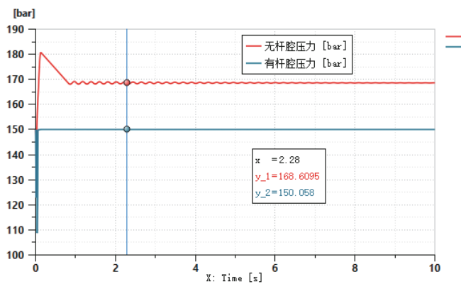
图8 液压缸无杆腔压力 2
