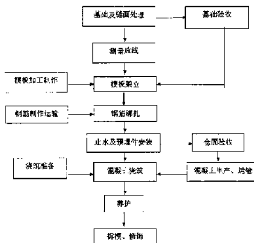
图1 混凝土浇筑工艺流程图
