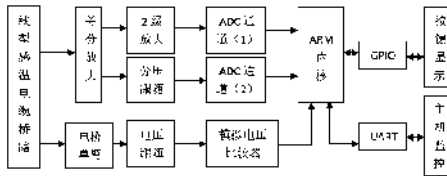
图 2-1 线型感温消防系统硬件框图
