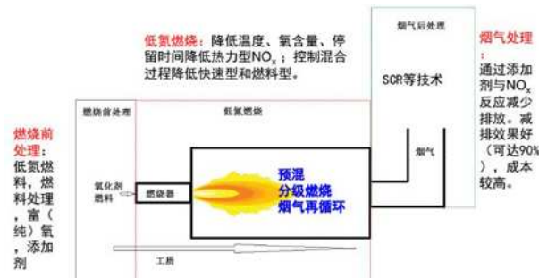
图2 低氮燃烧技术的应用流程
