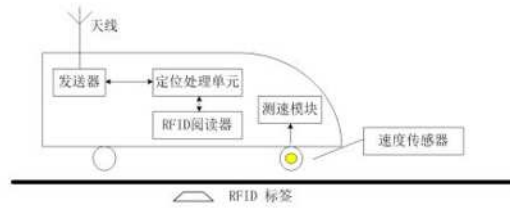
图2 RFID 机车定位系统结构图
