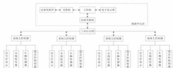
图1 “信集闭”系统总体结构
