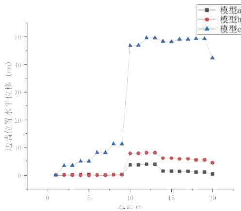
图5 边墙水平位移变化图
