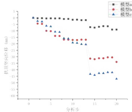
图 3 拱顶竖直位移变化图
