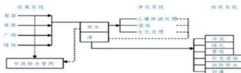
图1 建筑给排水设计中雨水利用流程图
