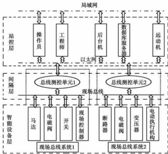
图1 电子信息工程自动化总线控制系统
