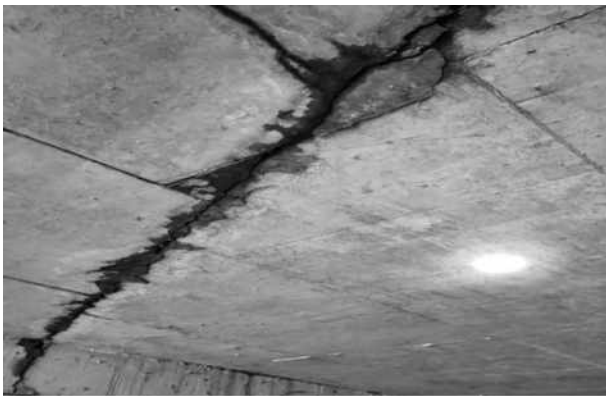
图1 桥梁横裂缝现象
