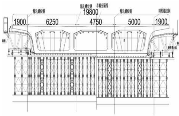
图 10 吊杆断面布置图
