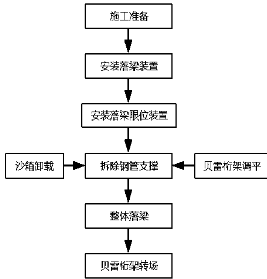
图3 工艺流程图
