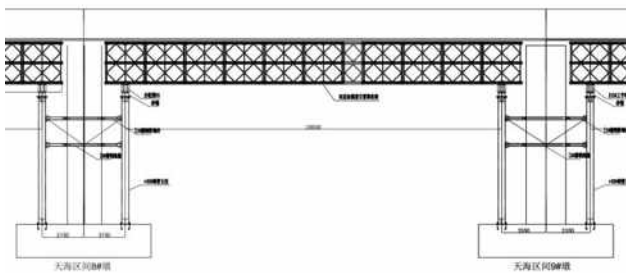
图 1 支架纵断面图（1 跨）
