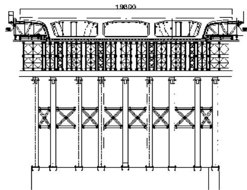
图 2 支架标准断面图
