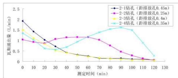
图 5 \Phi 94\text{mm} 钻孔排放半径考察钻孔涌出量衰减曲线
