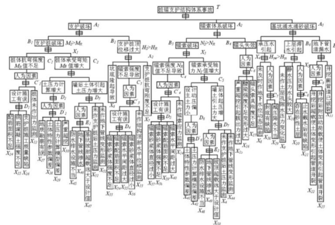
图1 桩锚支护结构体系事故树
