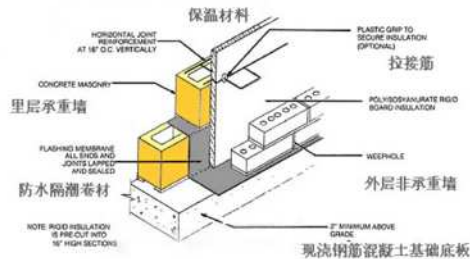
图1 外墙节能保温施工工艺
