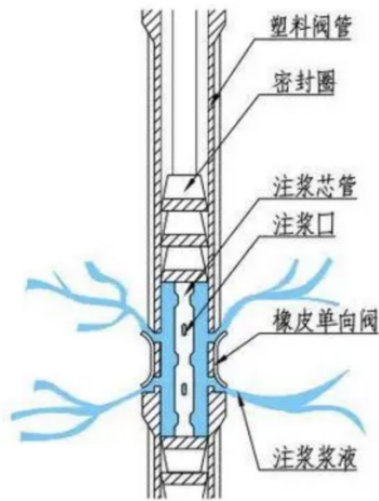
图4 袖阀管注浆原理图
