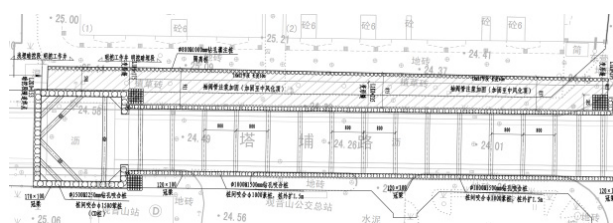
图2 塔埔社区袖阀管注浆平面布置图
