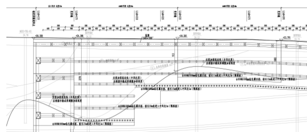
图3 塔埔社区袖阀管注浆纵断面布置图
