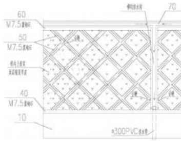
图3.2是亲水平台护岸结构的平面图
