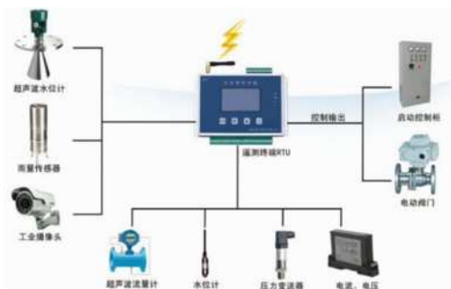
图2 水资源信息技术管理终端
