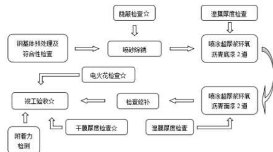
图1 压力钢管洞内防腐施工工序图
