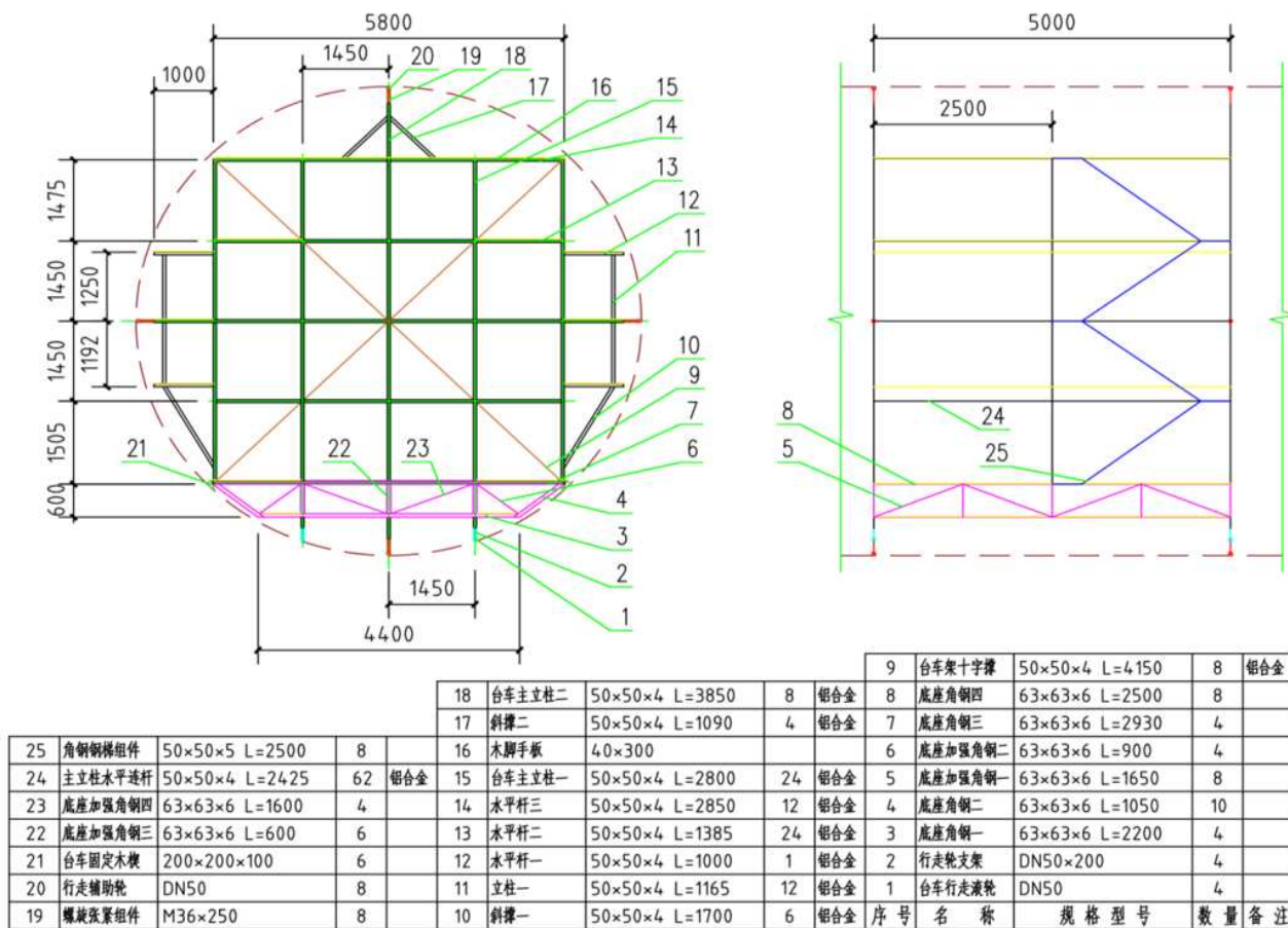
图3 防腐专用台车
