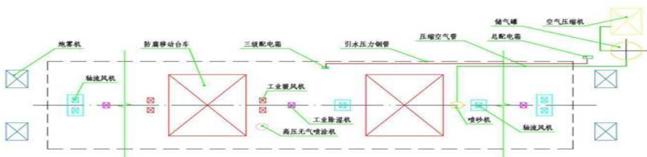
图2 引水压力钢管洞内防腐施工设备平面布置图
